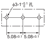
<印刷基板用端子孔加工图(参考)>
