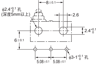
<印刷基板用端子孔加工图(参考)>
