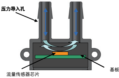
图 1 MEMS 差压传感器（D6F-PH）的内部剖面示意图
