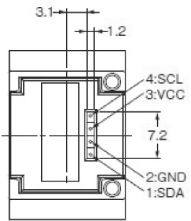
图 2 D6F-PH0505AD3 / D6F-PH0025AD1 / D6F-PH5050AD3 的外形尺寸图
