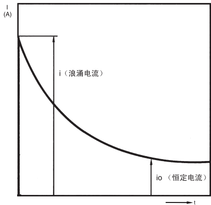
浪涌电流
