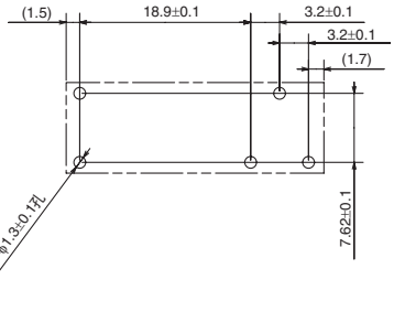
印刷基板加工尺寸 (BOTTOM VIEW)
