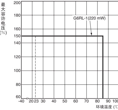
G6RL-1(A)-(4)-(ASI)-(PL) 环境温度和最大容许电压
