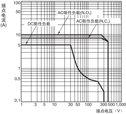
G6RL-1(A)-(ASI)-(PL) 开关容量的最大值
