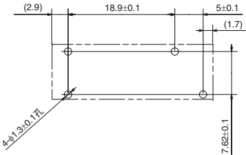
印刷基板加工尺寸 (BOTTOM VIEW)
