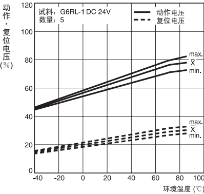
G6RL-1(A)(4) 环境温度和动作·复位电压
