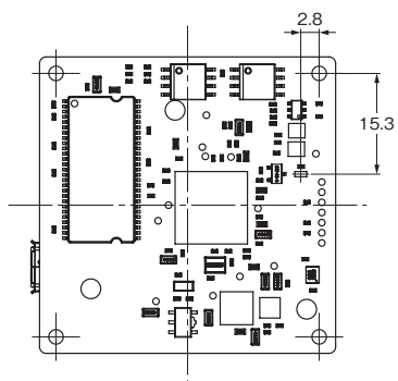
主基板背面
