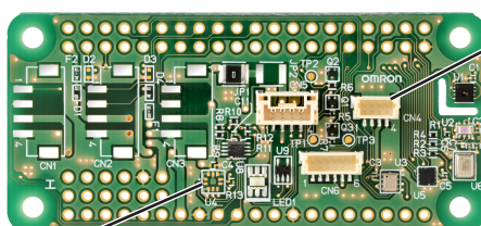
OMRON传感器评估板
