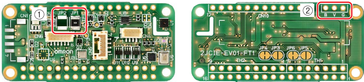
2JCIE-EV01-FT1 布局图
