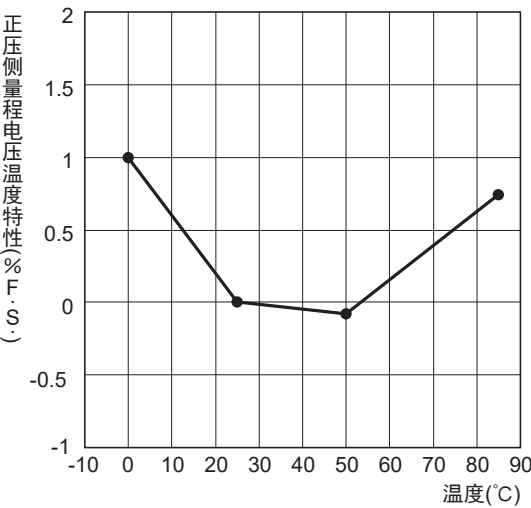
量程电压温度特性(0~50kPa)
