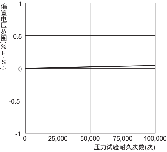
压力耐久试验(0~75kPa)
