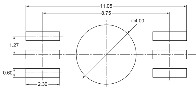
推荐基板加工尺寸
