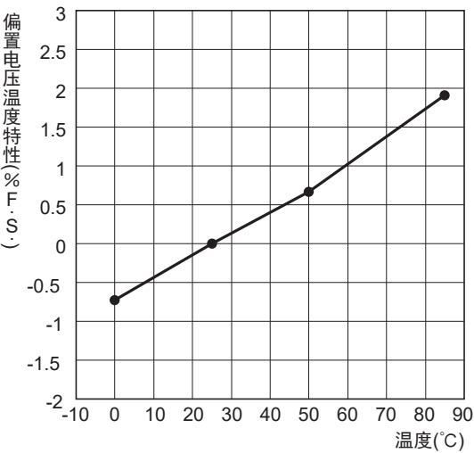
偏置电压温度特性(0kPa时)
