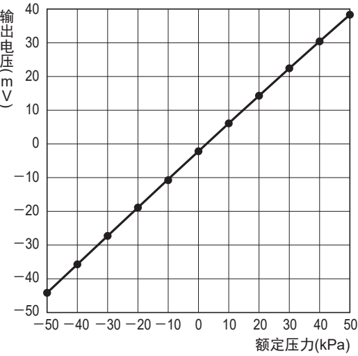
额定压力-输出电压
