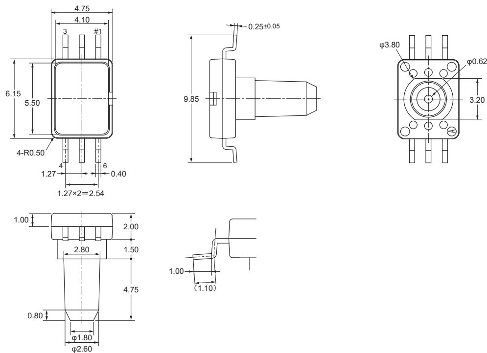
端子图 (传感器上表面)
