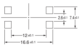
印刷基板焊盘尺寸示例 (TOP VIEW) (基板 t=1.6)
