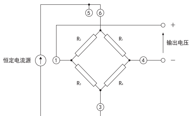
连接图
