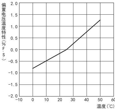
偏置电压温度特性
