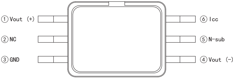
端子图 (传感器上表面)
