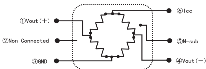
连接图
